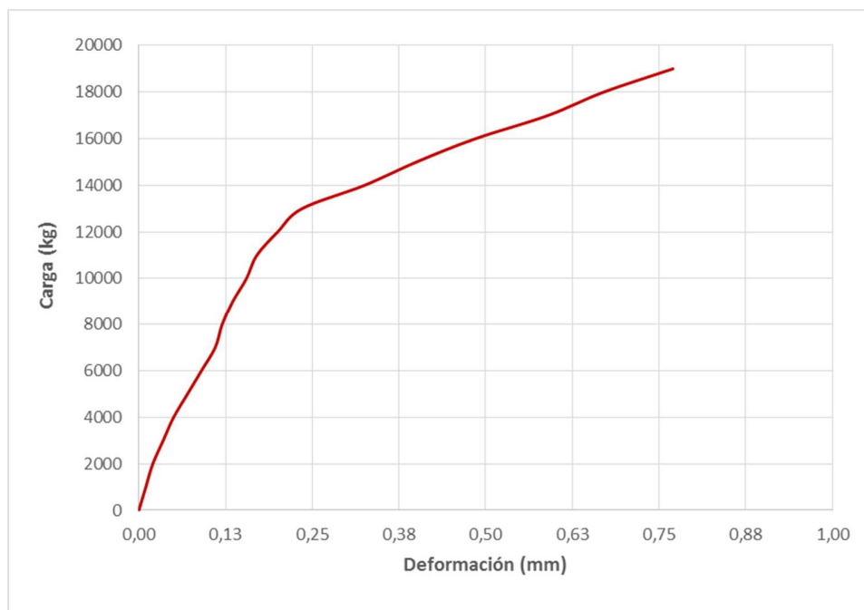
Figura 5 – Gráfico de carga-deformación en probeta 13
