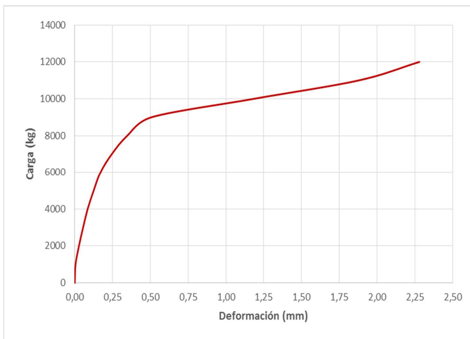
Figura 4 – Gráfico de carga-deformación en probeta 12
