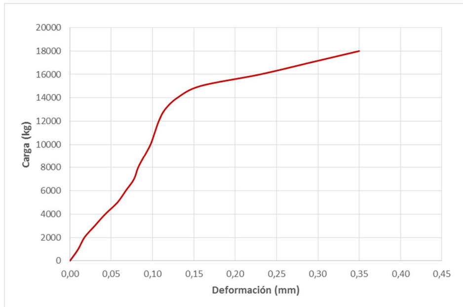
Figura 3 – Gráfico de carga-deformación en probeta 11
