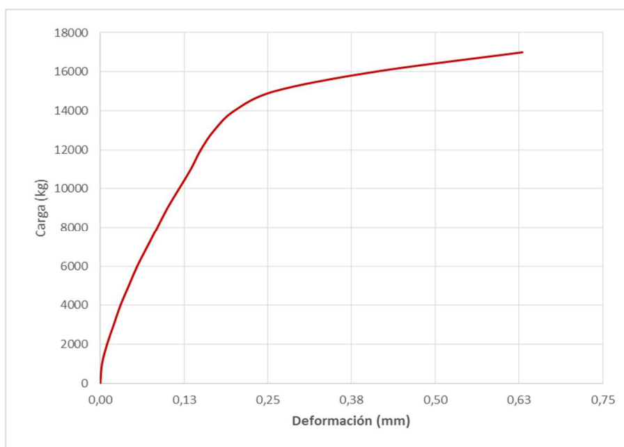
Figura 2 – Gráfico de carga-deformación en probeta 10
