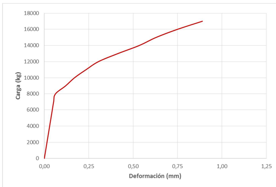
Figura 1 – Gráfico de carga-deformación en probeta 9
